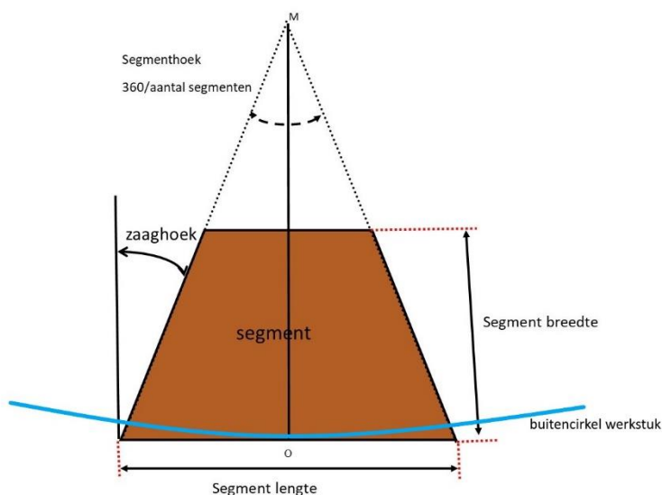
Figuur 10: het segment en zijn afmetingen
